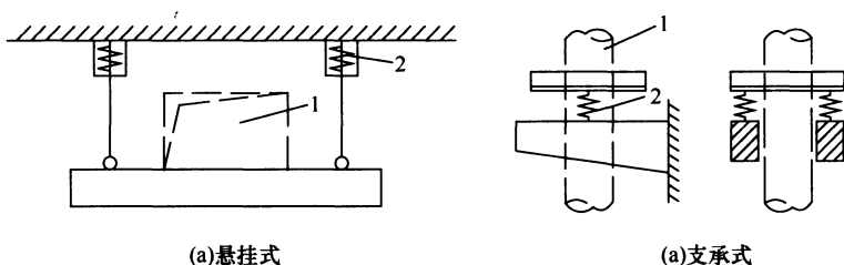
图 7.2.3-1 隔振方案
